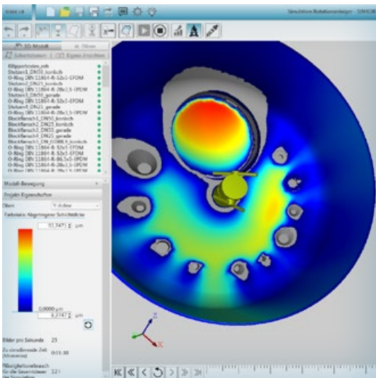
Abb. Neuartiges Reinigungssystem zur Realisierung intelligenter, bedarfsgerechter Reinigung. www.simkor.eu
